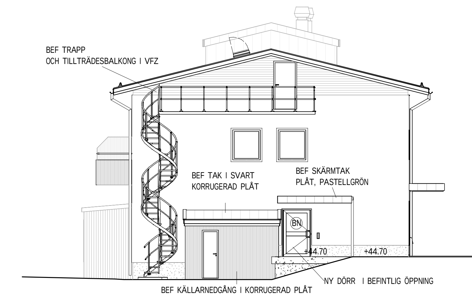
1/100 FASAD MOT NORDOST, PARKERING
