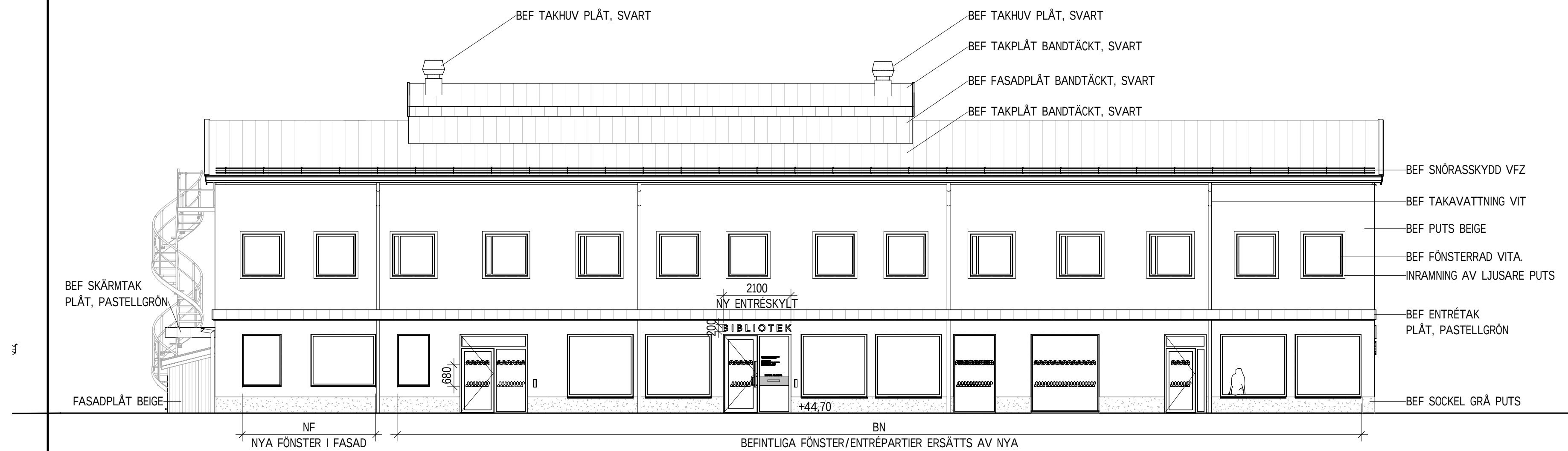
1/100 FASAD MOT NORDVÄST, ENTRÉSIDA
