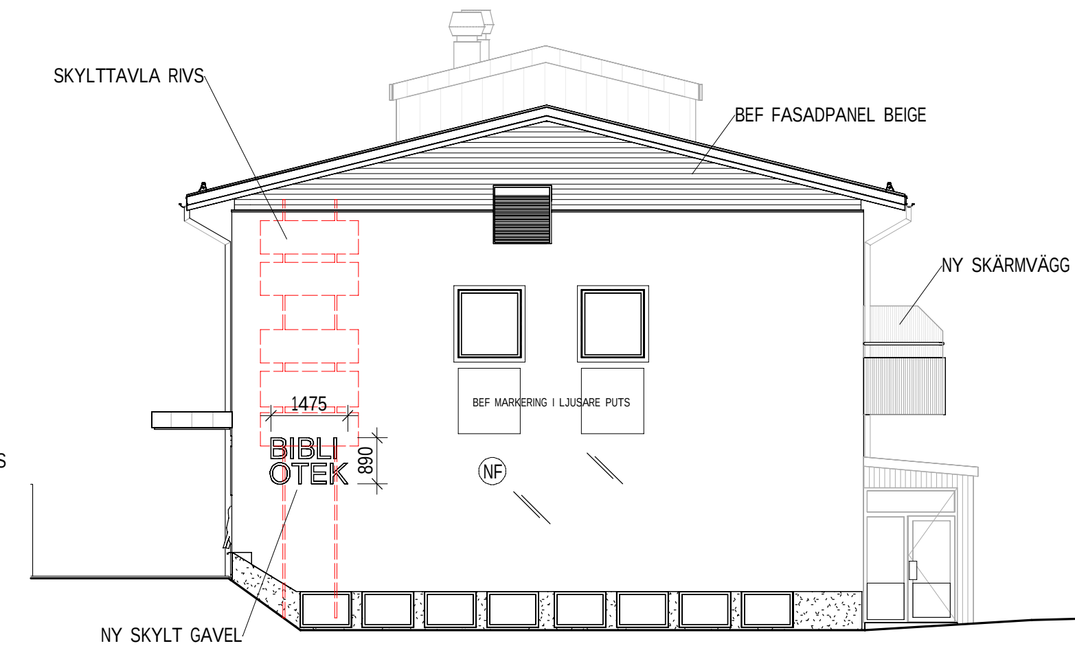
1/100 FASAD MOT SYDVÄST, STORGATAN
